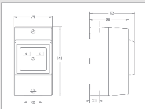
Gehäuse A
