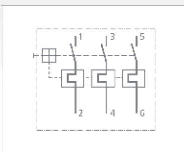
Motorschuttschalter OKN
