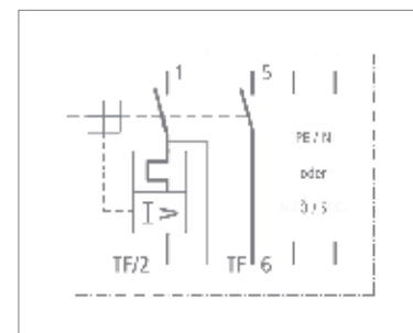
Motorschuttschalter TFE2 optional 15 und / oder 10
