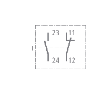
Hilfsschalter Hi 11 (15 / 10)
