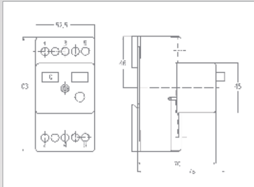
Motorschuttschalter OKE2 / MKE2
