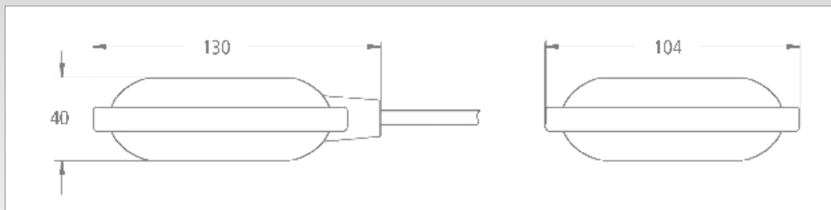
Schwimmerschalter PSN
