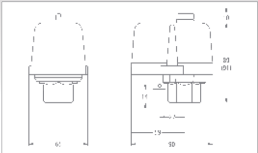
Druckschalter MDR-2
