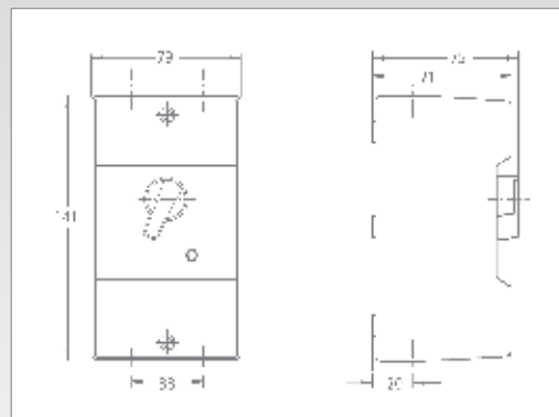
Gehäuse H
