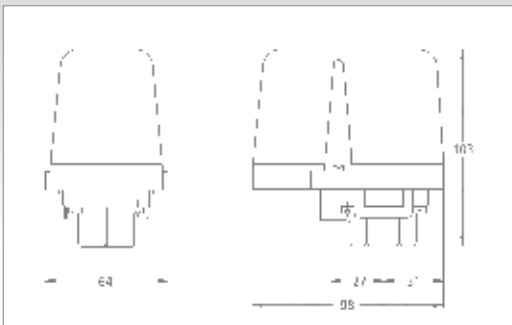
Druckschalter MDR 43
