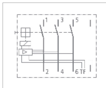
Motorschuttschalter TFA2
