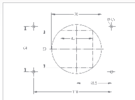
Einbau-Ausschnitt für Frontplatte E
