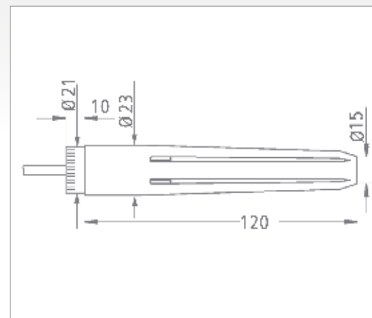
Tauchelektrode TEL...
