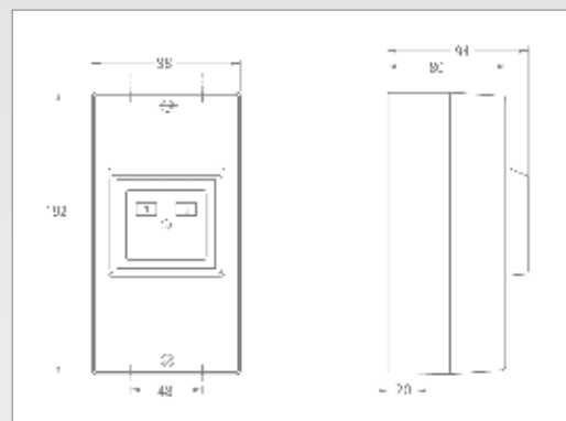
Gehäuse B
