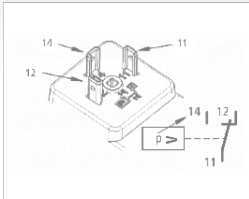
Standardausführung MDR-P
