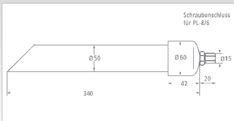
Tauchglocke OGL
