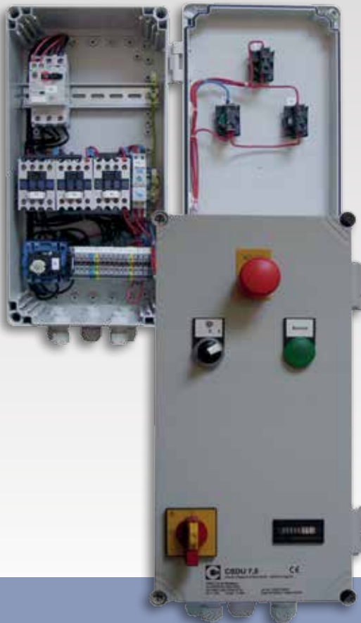
Abb. CSDU 7,5 komplett
