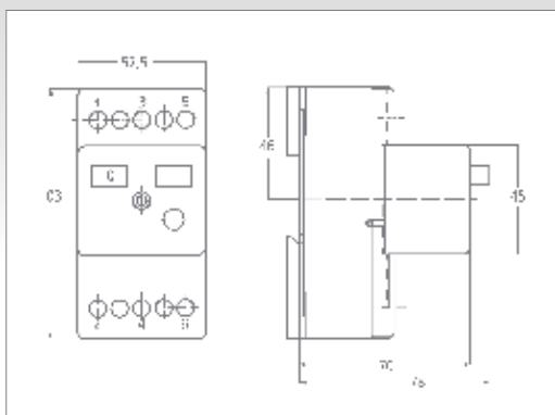
Motorschuttschalter TFE2 / TFA2
